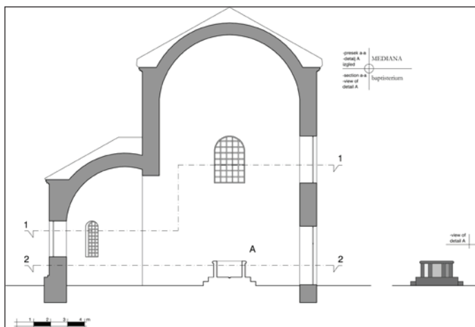
Сл. 31 Медијана, идеална реконструкција, подужни пресек са piscinom (арх. Е. Васић Петровић)
