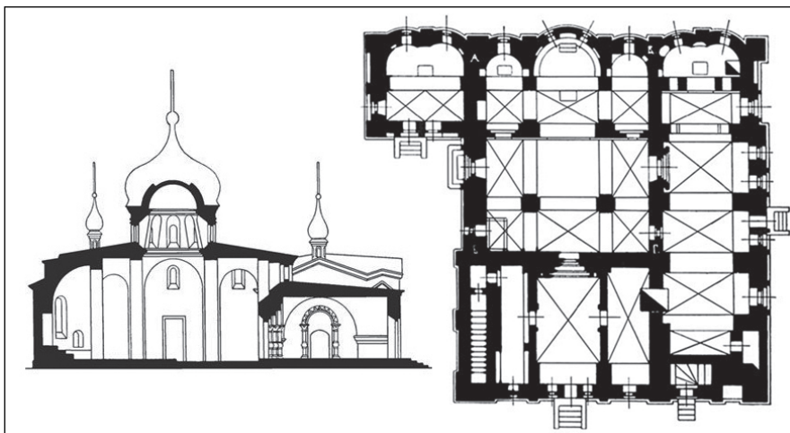
Сл. 3 Москва. Католикон Спаса на Бору, XIV-XVI в., план, пресек. Цртеж А.А. Мартинова, сред. XIX в.
