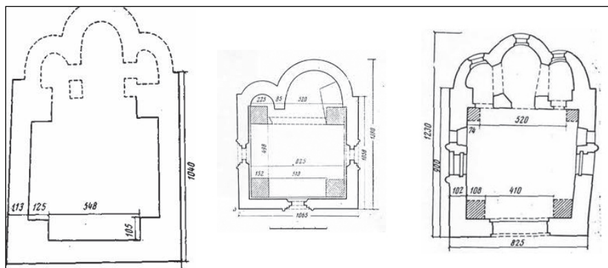
Сл. 9 Коломна, католикон Бобренева и Старо-Голутвина манастира, црква Зачећа Светог Јована Крститеља у Городишчу, планови XIV в.
