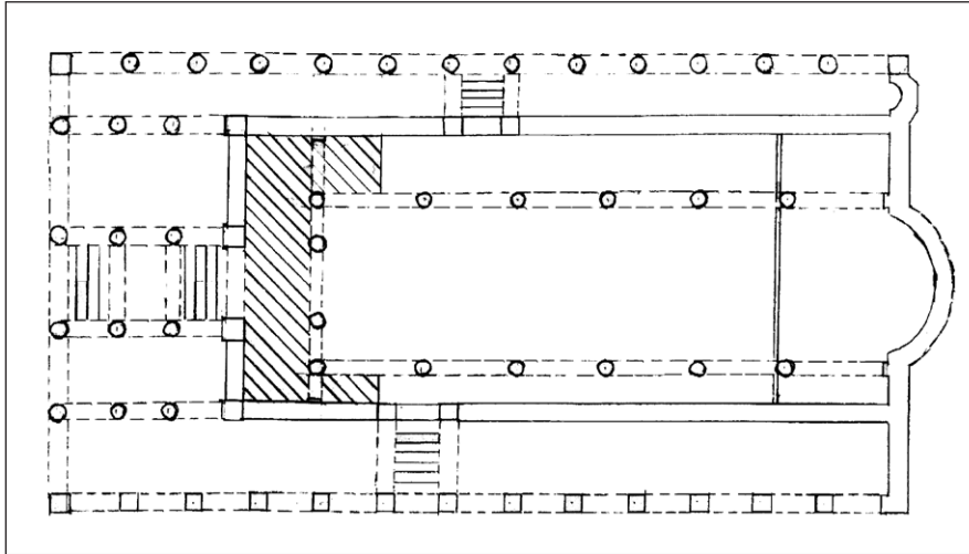
Sl. 3. Основа храма Св. Арханђела Михаила и Гаврила у Нишу Fig. 3. The base of the Church of Holy Archangels Michael and Gabriel in Niš
