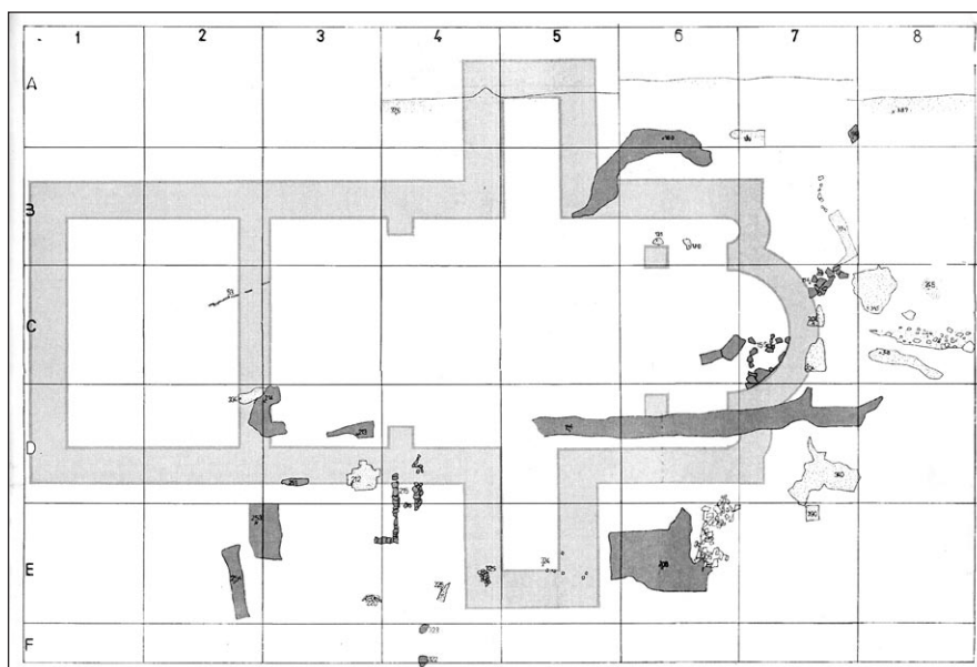
Сл. 4 Претпостављајући изглед основе Немањине цркве, према В. Корућу
