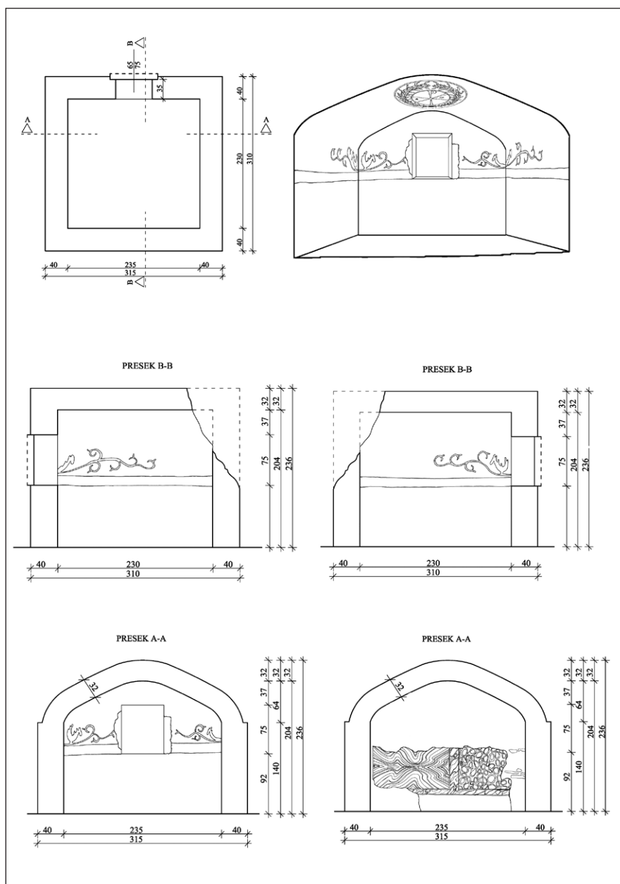
Сл. 10 Основа, изглед, подужни и попречни пресеци (арх. Ј. Ракоција и арх. М. Диманић)
