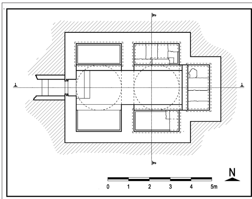
Сл. 15 Гробница бр. 19, основа, (арх. Ј. Ракоција)
