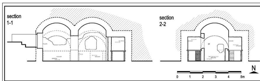
Сл. 16 Гробница бр. 19, подужни и попречни пресек, (арх. Ј. Ракоција)
