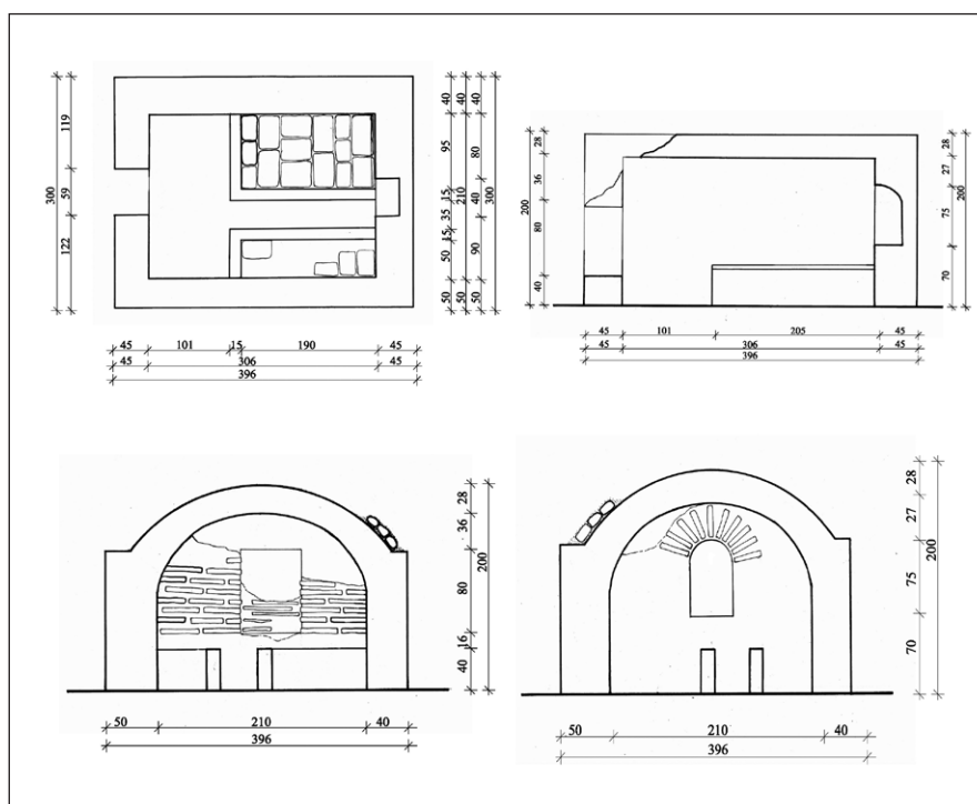
Сл. 21 Гробница у Топоници, основа, подужни и попречни пресеци (према арх. Ј. Ракоција и арх. М. Диманић)
