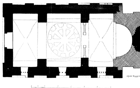
Сл. 18 Св. Петар у Прику код Омиша, основа
