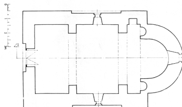
Сл. 30 Св. Никола у Шуменику, основа
