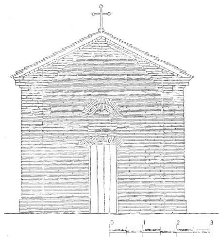
Сл. 8 Св. Јован у Орљану, изглед са запада
