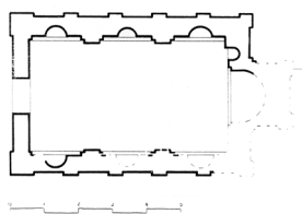
Сл. 22 Св. Тома у Кутима, основа и унутрашњи изглед
