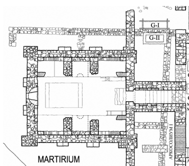
Сл. 24 Ниш, Мартиријум ранохришћанске базилике
