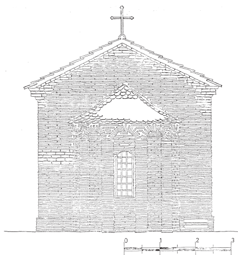
Сл. 7 Св. Јован у Орљану, изглед са истока
