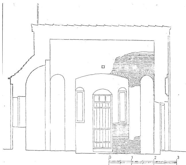
Сл. 9 Св. Јован у Орљану, подужни пресек
