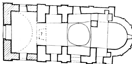
Сл. 28 Маркова црква, основа
