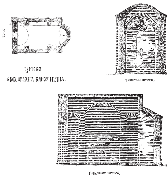
Сл. 5 М. Валтровић и Д. Милутиновић, основа и претпостављајући изглед цркве, 1878.
