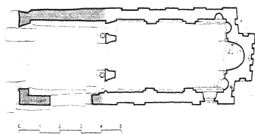
Сл. 21 Св. Димитрије у Габрилима, основа
