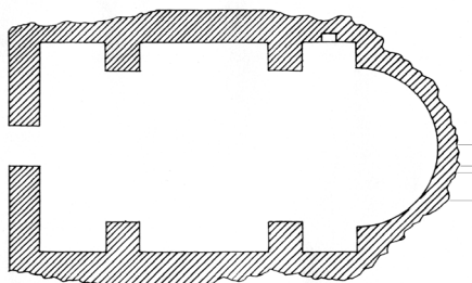
Сл. 29 Црква Кичавска, основа
