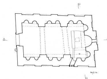
Сл. 23 Св. Иван Подата, основа
