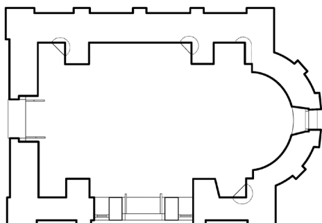
Сл. 10 Св. Јован у Орљану, основа
