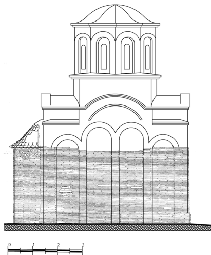
Сл. 32 Св. Јован у Орљану, идеална реконструкција, према арх. Јелена Ракоција.
